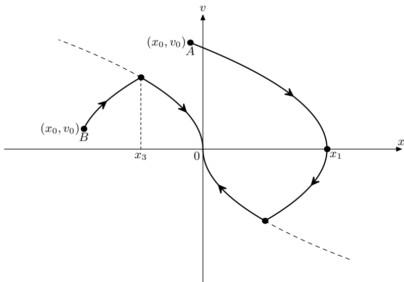
Obr. 1: Nákres situace. Všechny paraboly mají vrchol na ose x a jsou stejně zakřivené. Dělicí paraboly jsou čárkované, čáry se šipkami odpovídají nejrychlejším trajektoriím do počátku.
